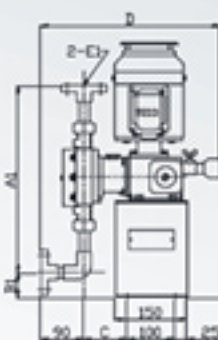
法蘭式
